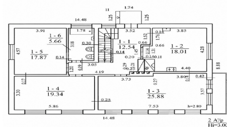
PIRMO AUKŠTO PLANAS
