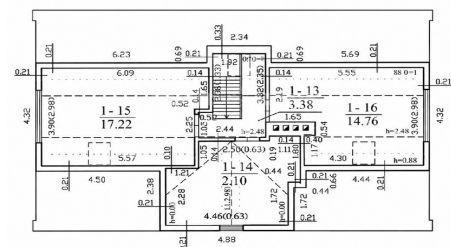
PASTOGĖS M1 PATALPŲ PLANAS
