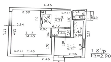
PIRMAS AUKŠTAS
