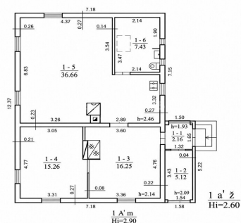
PIRMO AUKŠTO PLANAS
