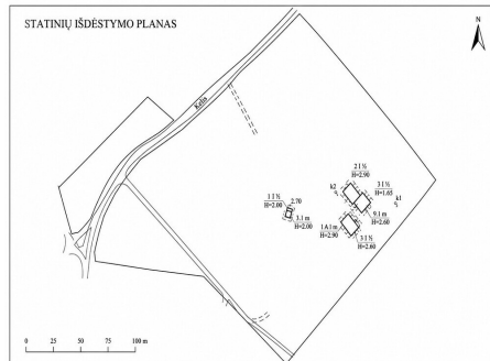
STATINIŲ IŠDĖSTYMO PLANAS
